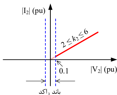
شکل ۷: مشخصه دامنه جریان راکتیو توالی منفی تزریقی نیروگاه تجدیدپذیر اینورتری نسبت به دامنه ولتاژ توالی منفی
