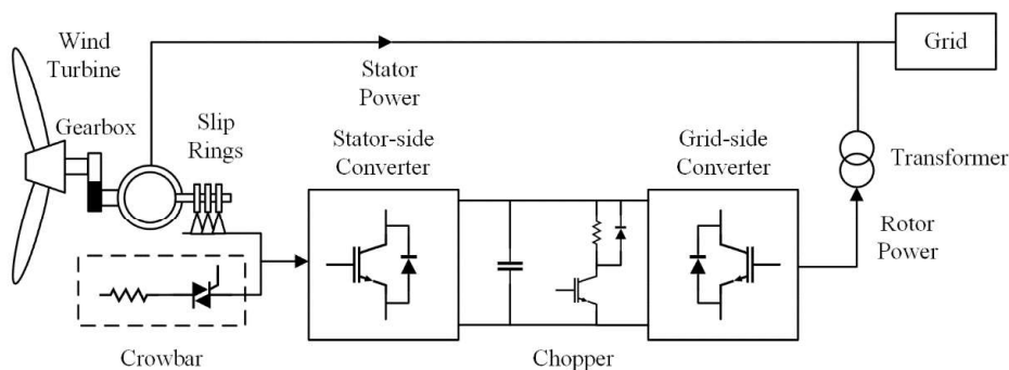
شکل ۲: ساختار نوعی نیروگاه بادی نوع ۳
