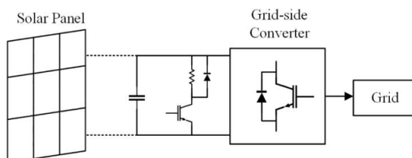
شکل ۱: ساختار نوعی نیروگاه خورشیدی فتوولتائیک
