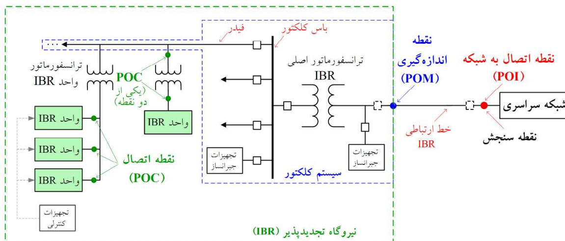
شکل ۴: نقاط POM، POI و POC در یک نیروگاه تجدیدپذیر اینورتری
